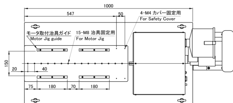
上面図
